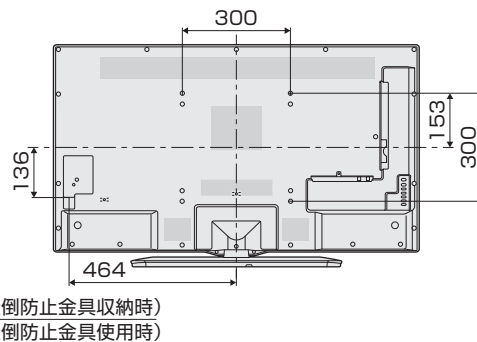
壁掛け金具取り付け部の寸法
